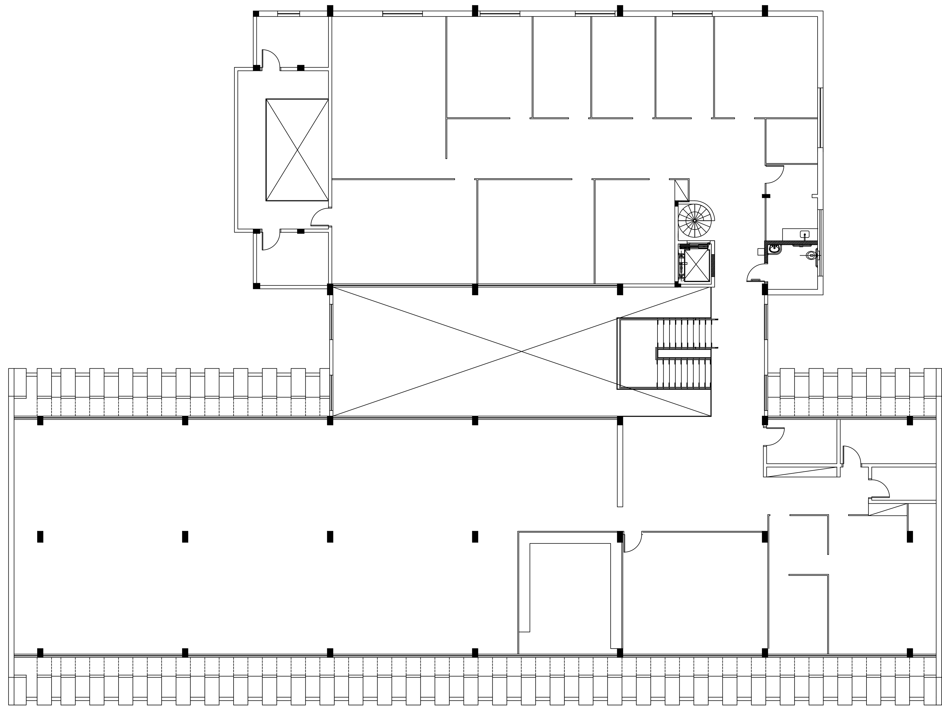
SEGUNDO PAVIMENTO 1:100
